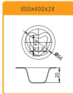
SN9214 Mini Heart Cake Mould-54 Indents (Silicone)
