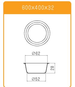
SN9088 35连布丁模(矽利康) 全包式
