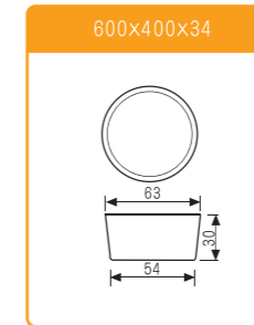
SN9084 28连布丁模(矽利康) 全包式
