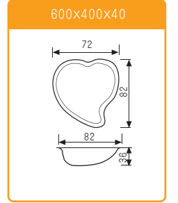
SN9023 28连桃型模(矽利康)
