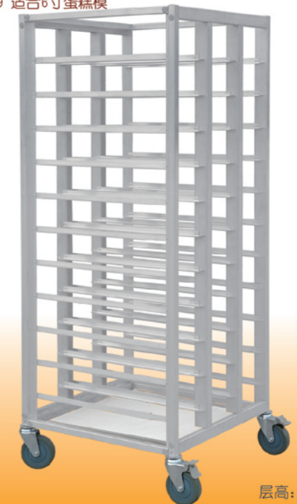
SN1993 11层组合式蛋糕模冷却车(阳极) 809x750x1695
