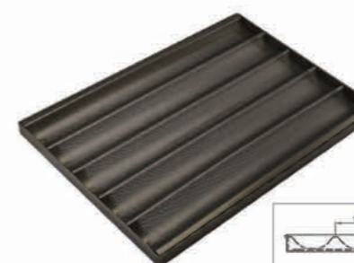
SN1593 ¥ 7,400 5連フランスパン天板(ノンスティック1000) アルミ合金 660x460x33
