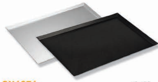
SN1071 ¥3,100 アルミ合金天板 (アルマイト) 1.5mmアルミ合金 600x400x20
